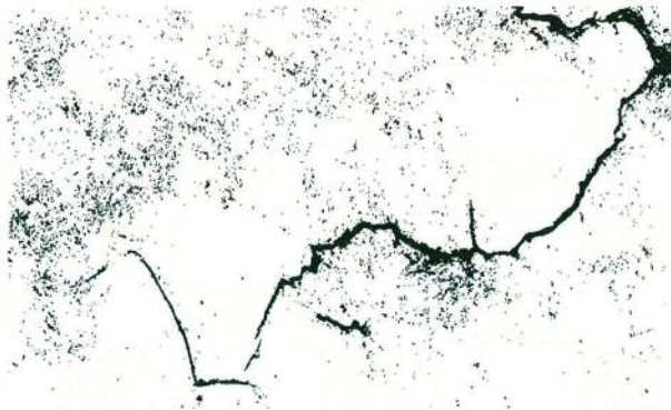
溶接構造用圧延鋼材の 溶接ポイント部に発生した遅れ割れ
